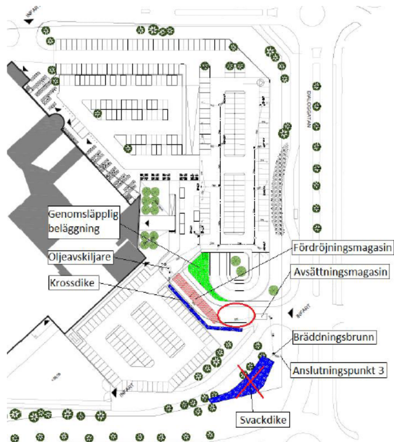
Dagvattenutredning 2017-01-24 (Novamark) Bilaga 4, Utredningsskiss alternativ 2. Placering för fler magasinrör är inringat i rött.
