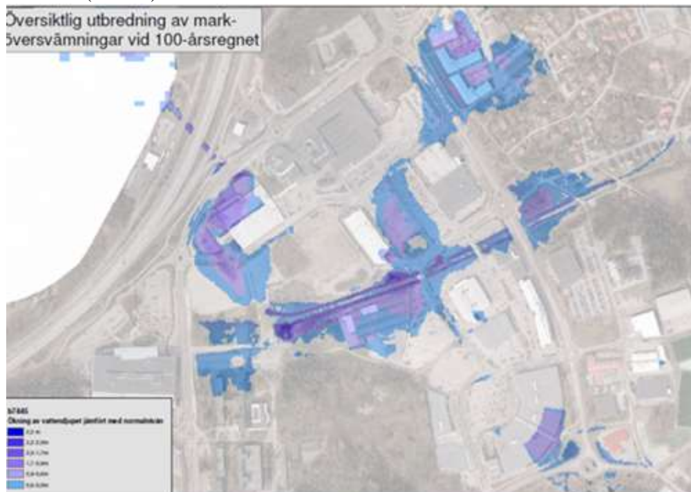
Stockholm Vatten ABs översiktliga beräkning av 100-års regn inom området
